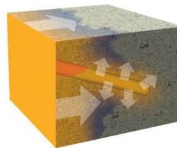
3) 使用PENETRON澎内传防水涂料 (PNC401) 涂覆墙面。新晶体会快速在墙壁的内部和外部同时生成。
