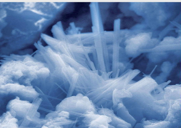
PENETRON 澎内传中的活性成分催化混凝土中的水泥水化产物反应后形成的结晶体照片，这些晶体结构可填充和封堵宽度达 0.5mm 的裂纹、孔洞和空隙。（放大倍数5000x）
